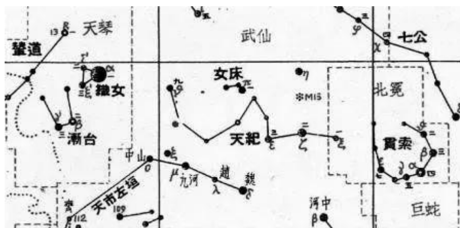
织女和贯索
