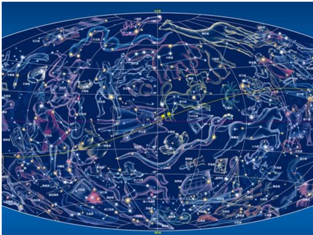
通用 88 星座
