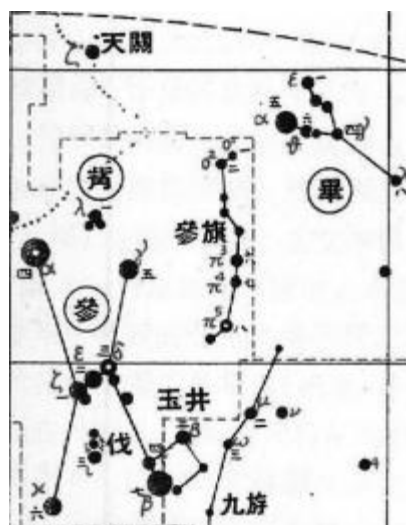
参宿与天关
